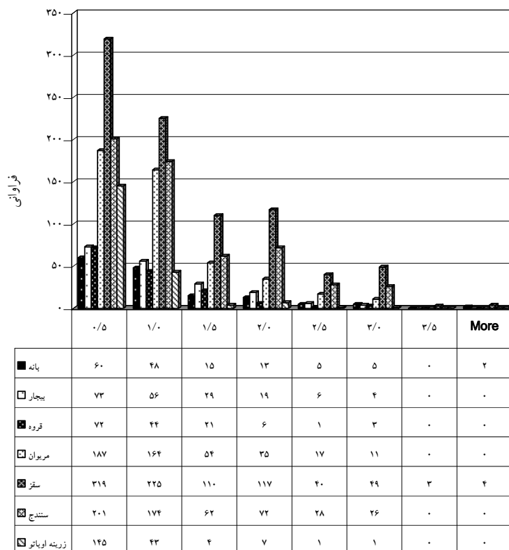
شکل ۱: فرآوانی ریزش برف غیر رگباری دردهماهای بیش از صفر درجه سلسیوس، در ایستگاه‌های استان کردستان، طی دوره آماری موجود.
