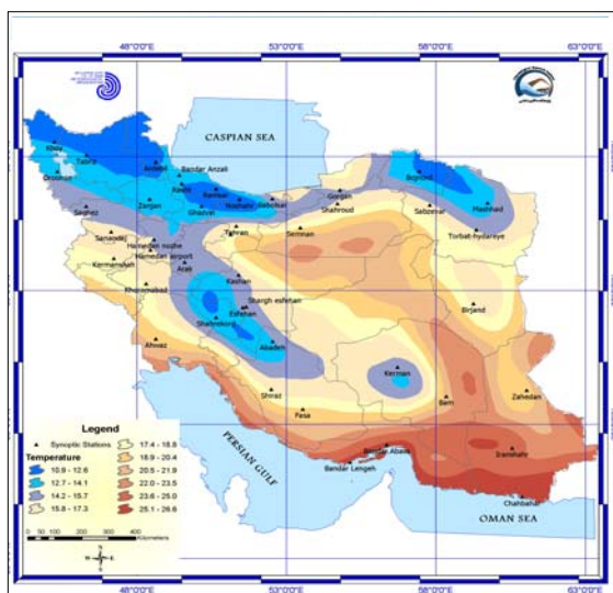
شکل ۱۳. توزیع مکانی میانگین دما در مدل MAGICC SCENGEN با داده‌های HADCM2
