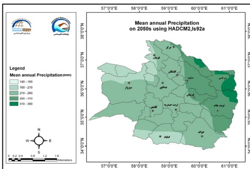
شکل ۹- توزیع مکانی میانگین بارش در مدل MAGICC SCENGEN با داده‌های HadCM2 با استفاده از سناریوی IS92A برای دهه ۲۰۵۰ استان خراسان رضوی
