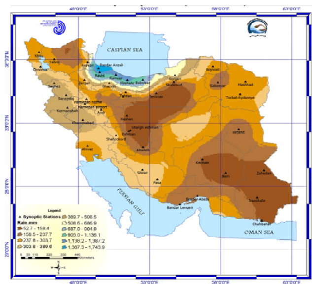
شکل ۴ - توزیع مکانی میانگین بارش در دوره آماری ۱۹۹۰-۱۹۶۱ میلادی
