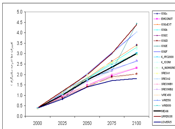
شکل ۱۲. برآورد تغییرات دمای دهه‌ای دمای کشور توسط مدل M-S با استفاده از داده‌های مدل گردش
