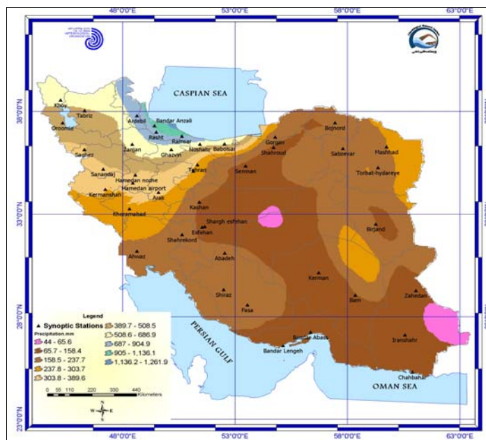
شکل ۶. بر آورد تغییرات دهه‌ای بارش در دوره ۲۰۰۰-۲۱۰۰ کشور توسط مدل M-S با استفاده از داده‌های مدل گردش عمومی جو ECHAM4
