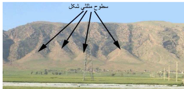
شکل ۹) نمونه ای از سطوح مثلثی شکل در دامنه جنوب غربی طاقدیس دنه خشک
