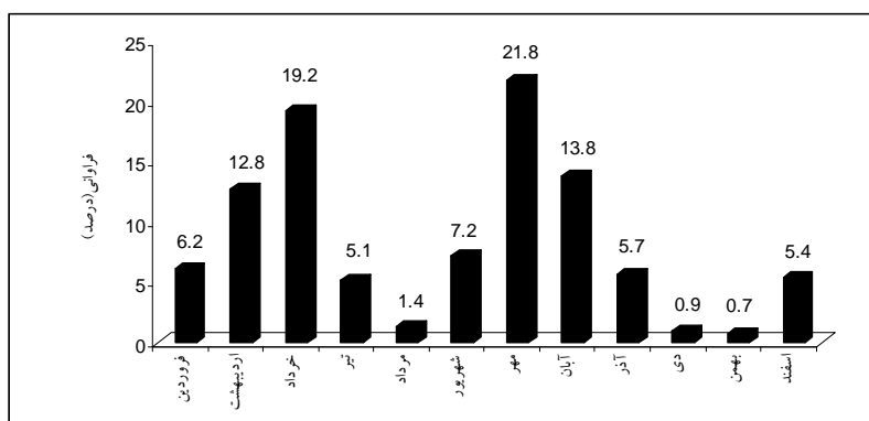
شکل ۷) وضعیت ماهانه آسایش اقلیمی ایستگاه قروه براساس شاخص SET*
