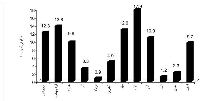
شکل ۳) وضعیت ماهانه آسایش اقلیمی ایستگاه سقز براساس شاخص SET*
