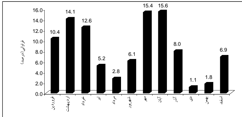
شکل ۱۵) وضعیت ماهانه آسایش اقلیمی استان کردستان براساس شاخص *SET
