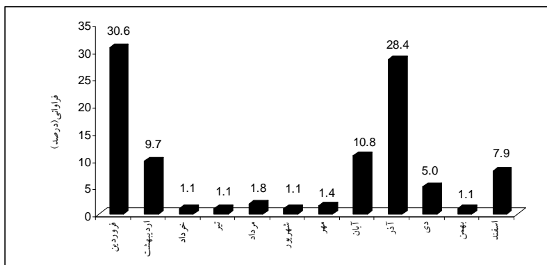
شکل ۱۴) وضعیت ماهانه آسایش اقلیمی ایستگاه بانه براساس شاخص PET
