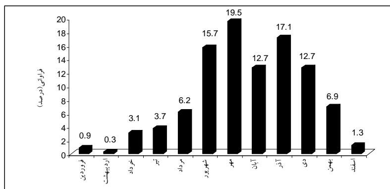
شکل ۱۰) وضعیت ماهانه آسایش اقلیمی ایستگاه زرینه براساس شاخص PET
