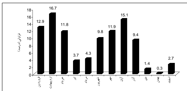
شکل ۴) وضعیت ماهانه آسایش اقلیمی ایستگاه سقز براساس شاخص PET
