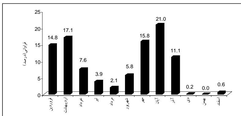
شکل ۱۲) وضعیت ماهانه آسایش اقلیمی ایستگاه مریوان براساس شاخص PET
