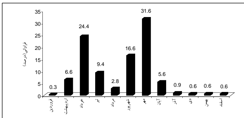
شکل ۱۳) وضعیت ماهانه آسایش اقلیمی ایستگاه بانه براساس شاخص SET*
