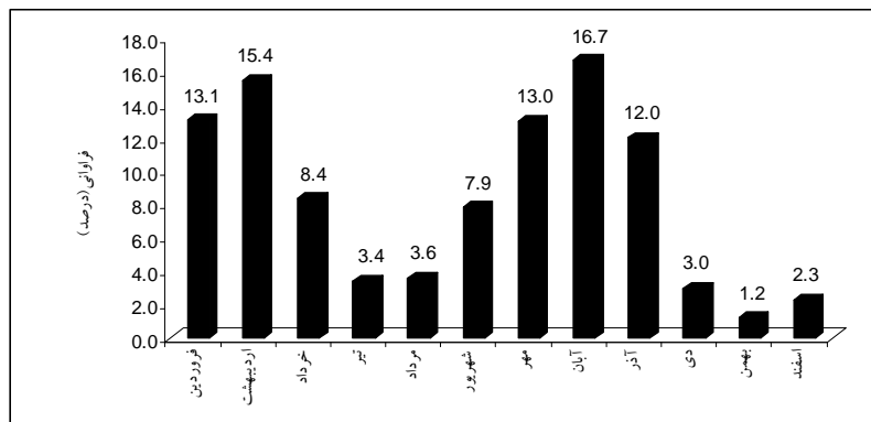
شکل ۱۶) وضعیت ماهانه آسایش اقلیمی استان کردستان براساس شاخص PET
