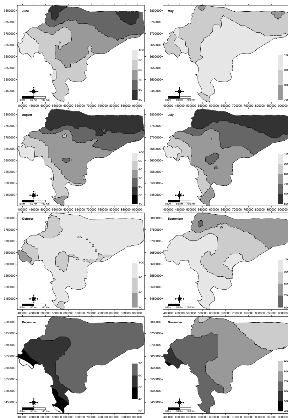
شکل (۳) نقشه پراکندگی شاخص آسایش گردشگری استان اصفهان در ماه‌های سال
