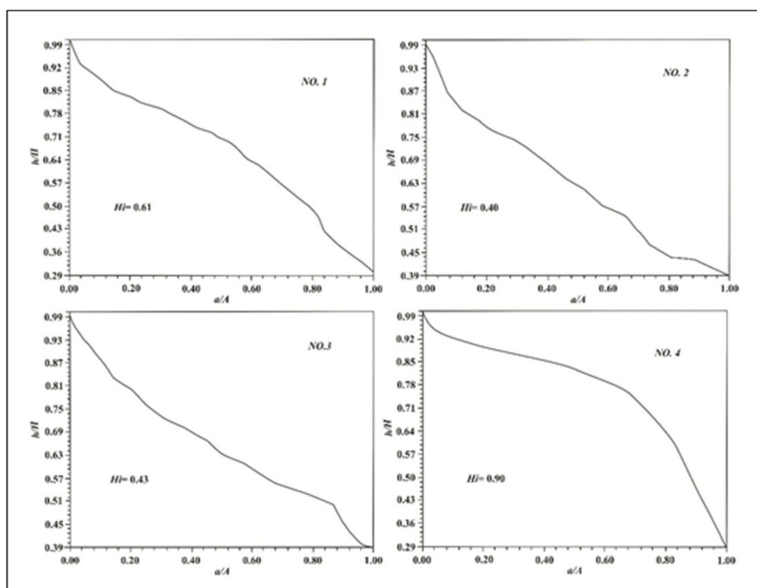
شکل ۶) منحنی‌های فرازسنجی زیرحوضه‌های رودخانه زیارت
