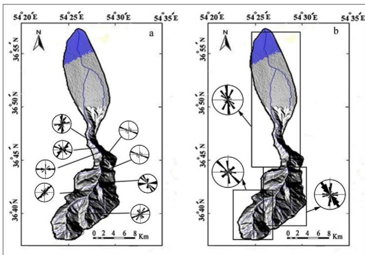
شکل ۸) نمودار گل‌سرخ شکستگی‌ها (a) و رودخانه‌ها (b) در حوضه زیارت
